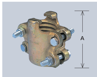
Material : Malleable 材 質：FCMB (可鍛鑄鉄) メッキ：ユニクロ 用 途：スチームホース 中圧ホース
