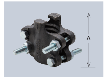
サイズ A 適用ホース外径： 1 78 40.0~46.0
