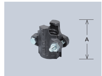
サイズ A 適用ホース外径： ½ 45 22.0~28.0 ¾ 70 33.0~37.0
